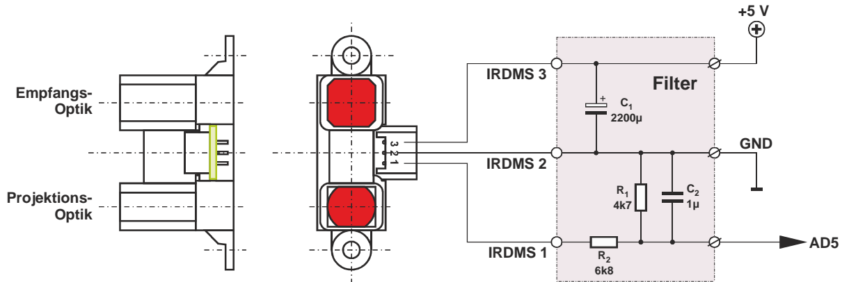
GP2Y0A02YK0F SHARP-IRDMS für den Messbereich 20 bis 150 cm
