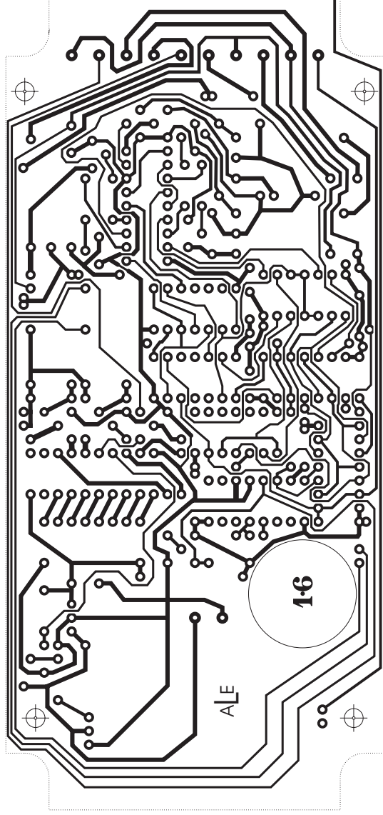
Lötseite
